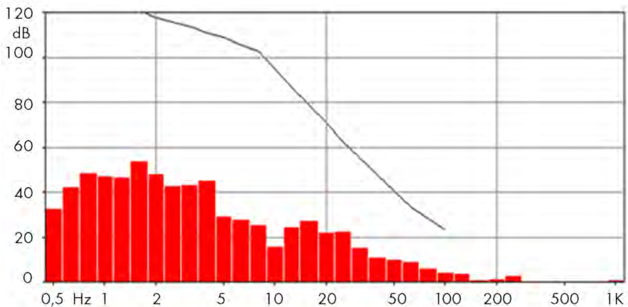
Abbildung 27: Terzspektrum des Ruhegeräuschs im Versuchsraum
